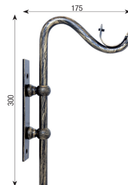
Mensola cigno singola aperta Ø35
